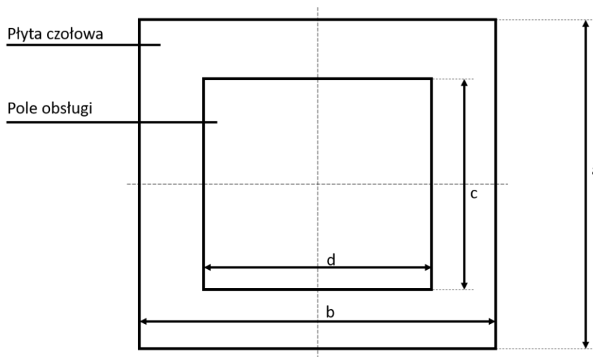
Ryc. 1. Wymiary przycisku przeciwpożarowego wyłącznika prądu
