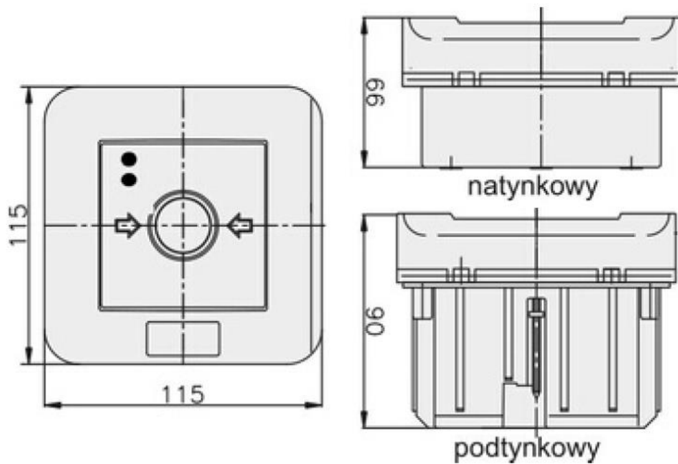
Ryc. 1. Wymiary główne ręcznego przycisku przeciwpożarowego wyłącznika prądu typu PPWP Źródło: Materiały producenta.
